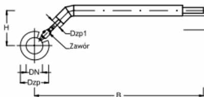
Kołano odgałęźne
