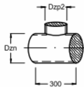
Trójnik TPG
